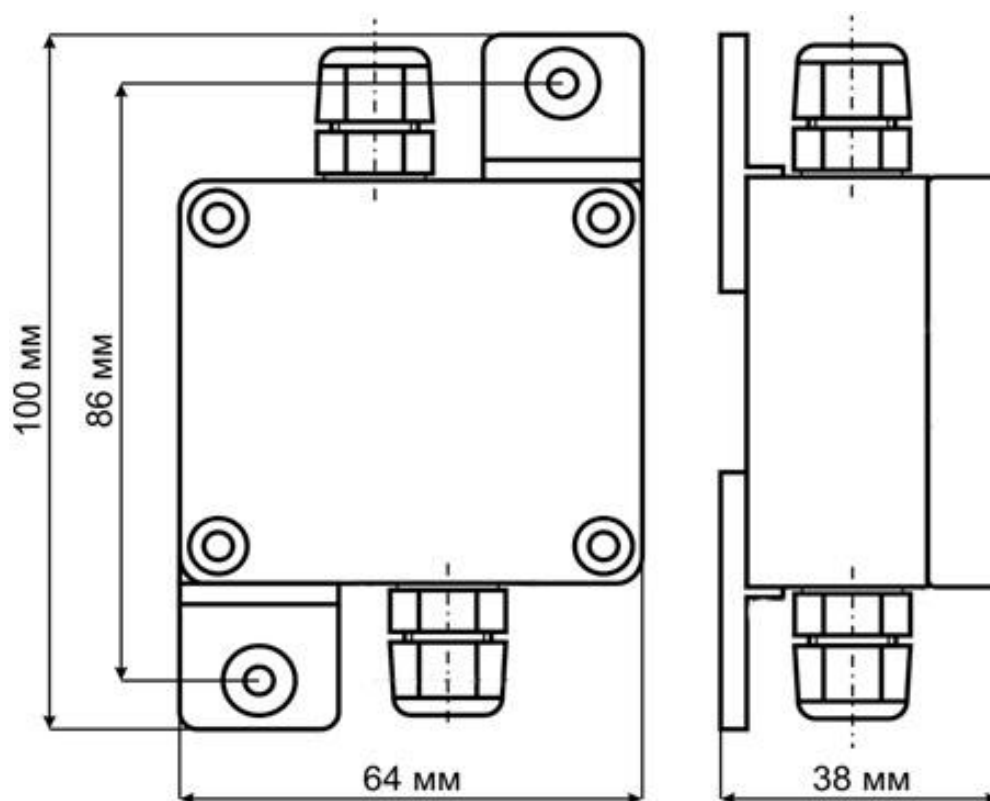
Рисунок А.4 – Тензопреобразователь (ТП)
