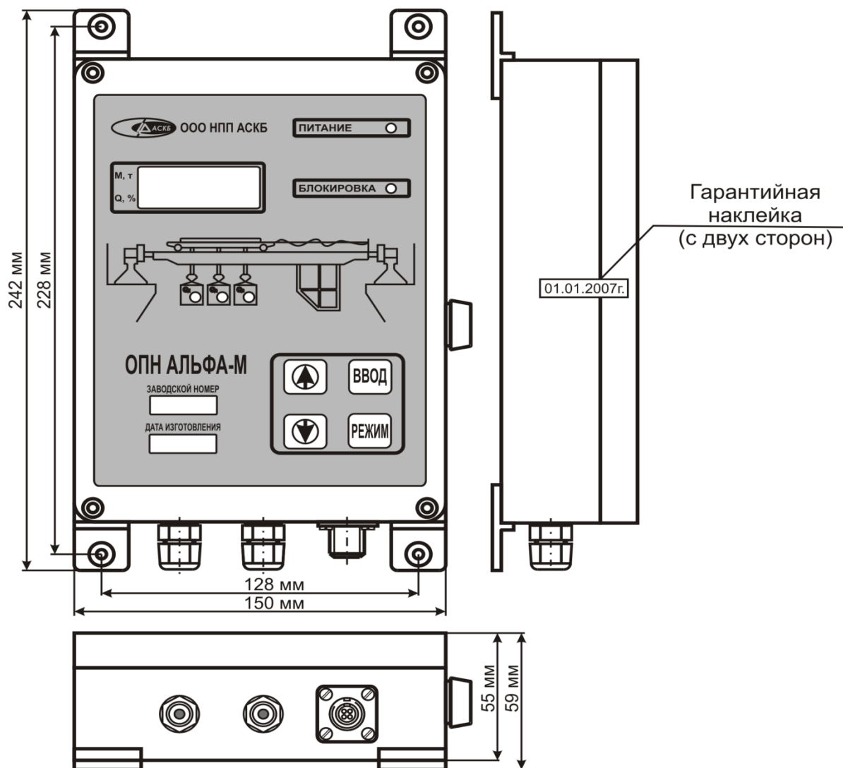
Рисунок А.1 – Бортовой микропроцессорный контроллер (БМК-01, -02, -03)
