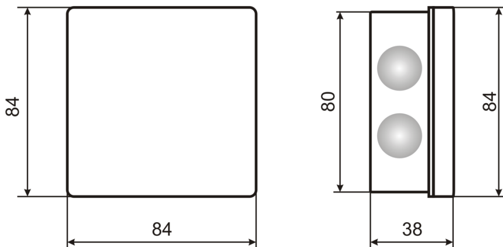
Рисунок А.3 – Блок зажимов (БЗ)
