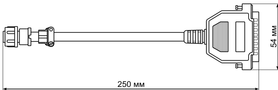
Рисунок А.2 – Прибор считывания (ПС)
